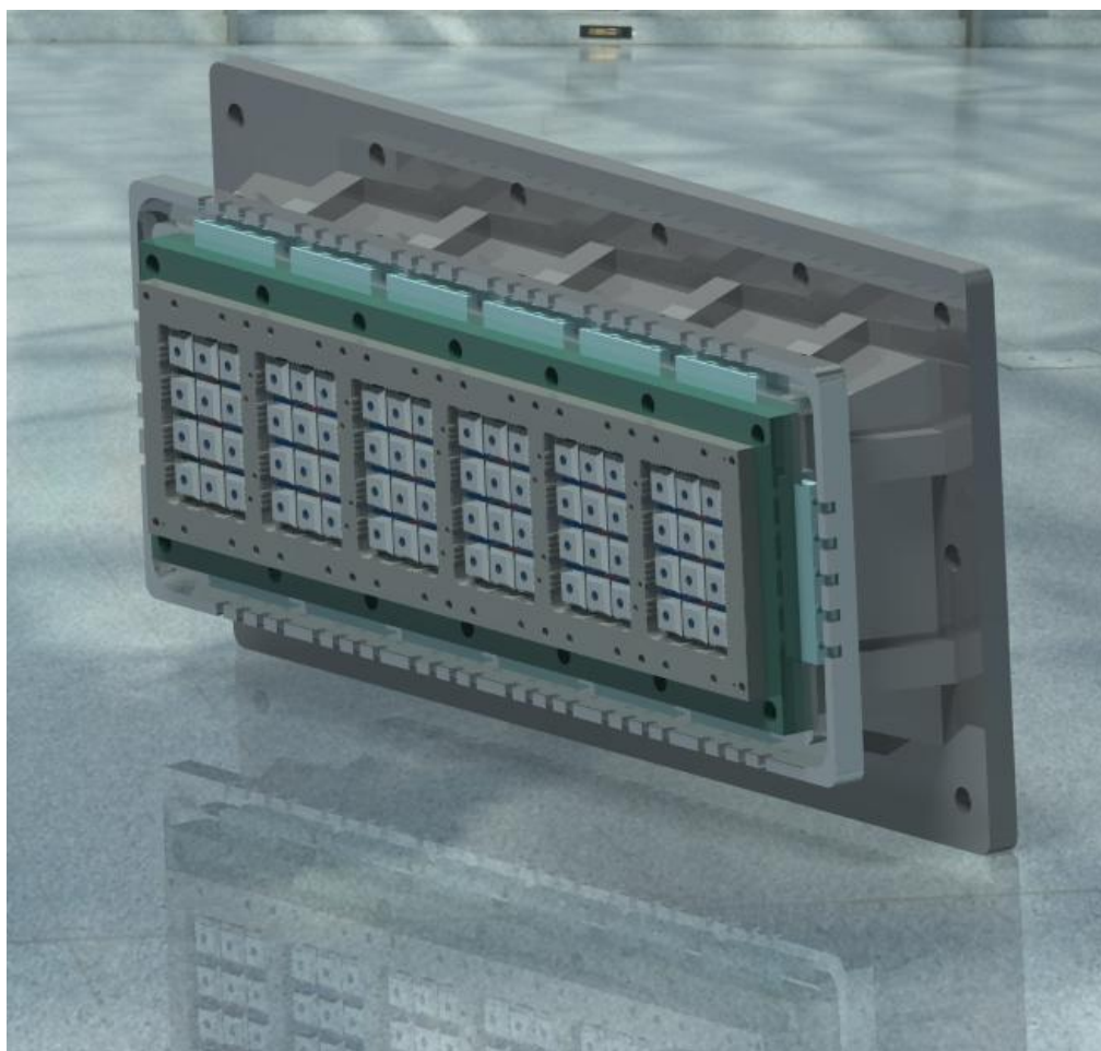
Conception de la filière 6 Sorties CF2 FC sur CATIA V5 R19
